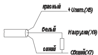
Схема подключения датчика PNP
