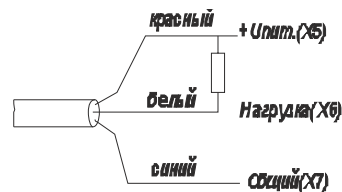
Схема подключения датчика NPN
